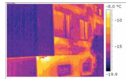
Ściany szczytowe budynków wielkopłytowych z widocznym wpływem zainstalowanego systemu ociepleń ETICS na intensywność wpływu ciepła
