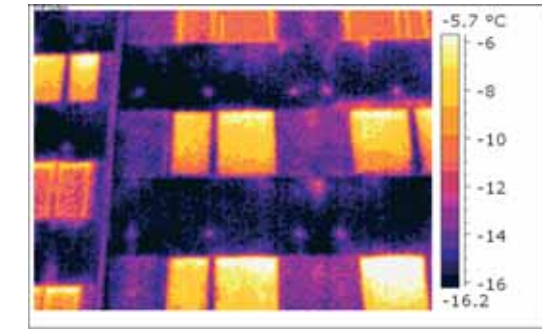
Ściana trójwarstwowa budynku wielkopłytowego z widocznym intensywnym wpływem ciepła przez łączniki międzywarstwowe
