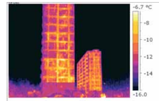
Ściana trójwarstwowa budynku wielkopłytowego z widocznym intensywnym wpływem ciepła przez węzły konstrukcyjne
