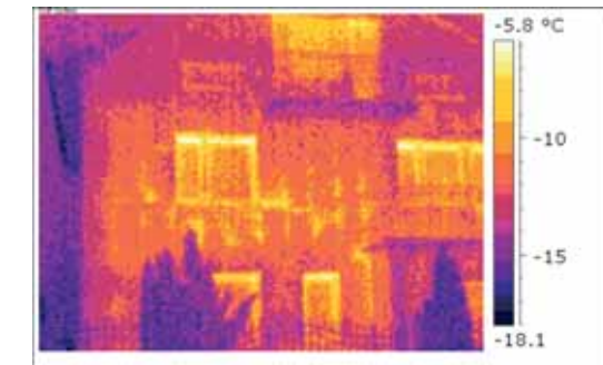
Ściana dwuwarstwowa z ociepleniem wykonanym w technologii suchej z widocznym intensywnym wpływem ciepła spowodowanym przepływem powietrza przez warstwę izolatora – nieskuteczna wiatroizolacja
