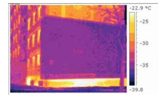
Ściany szczytowe budynków wielkopłytowych z widocznym wpływem zainstalowanego systemu ociepleń ETICS na intensywność wpływu ciepła
