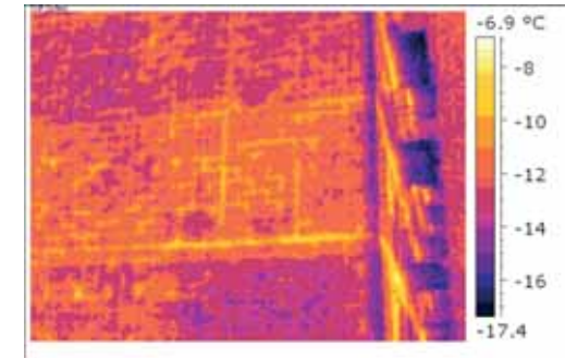
Ściana jednowarstwowa z bloczków betonu komórkowego z widocznym intensywnym wpływem ciepła przez spoiny
